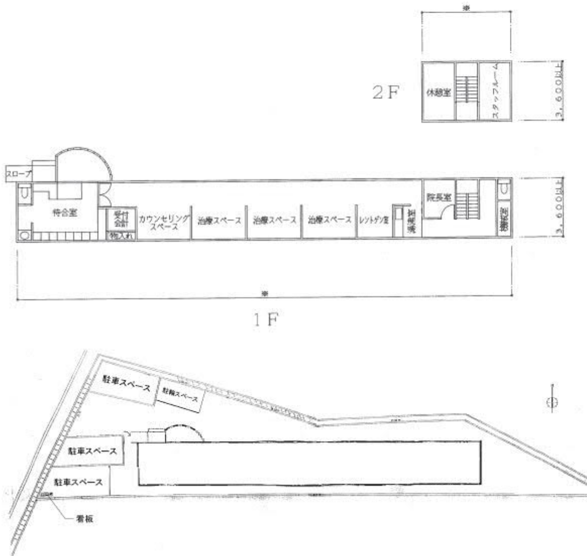
配置図
