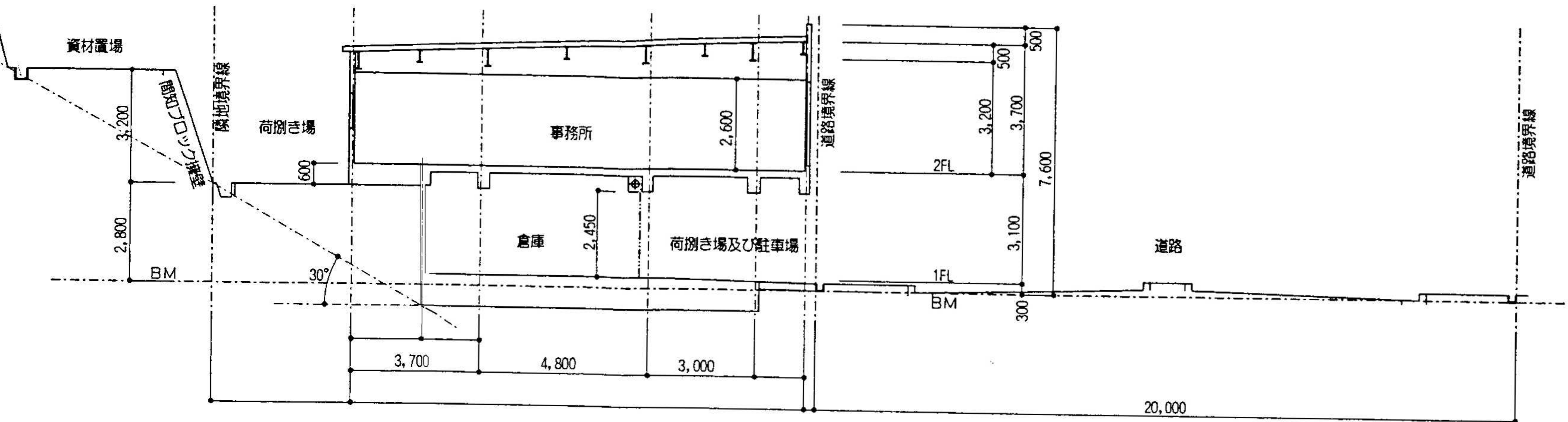
A-A 断面図 1:200
